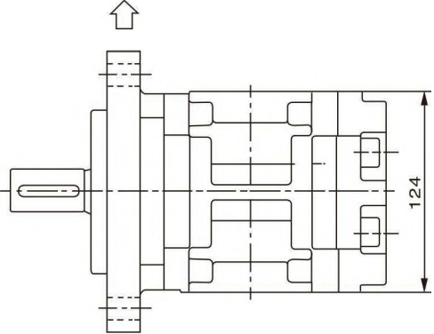
K1P法蘭 K1P Flange
